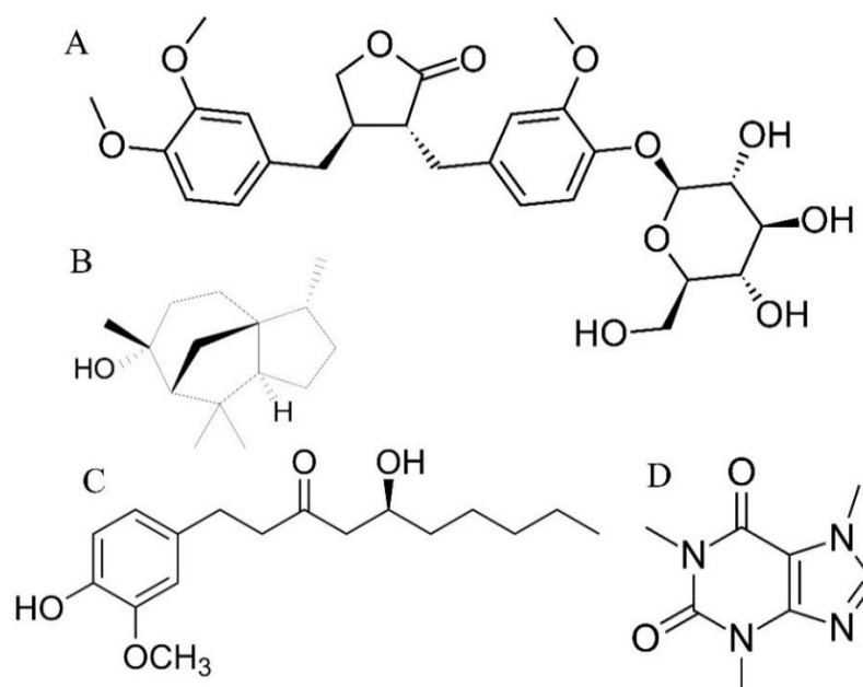
Fig. 4. Structural formulas of: arctiin (A), cedrol (B), 6-gingerol (C), and caffeine (D)
